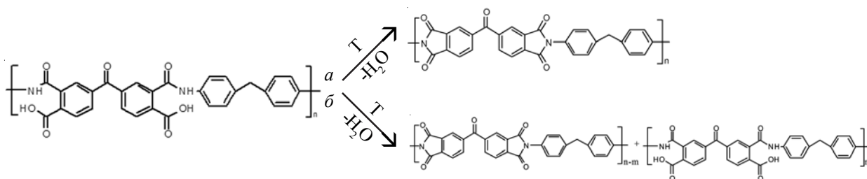
Рис. 2. Схема реакции имидизации ПАК при получении ПИ
