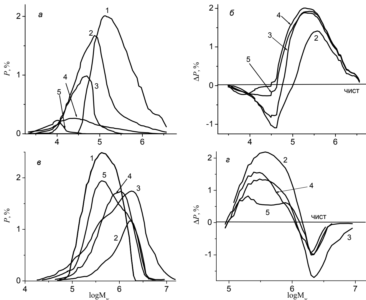
Рис. 4. ММР и \Delta P ПУ (а, б) и ПММА (в, г), полученных in situ из общей реакционной смеси при соотношении компонентов ПУ:ПММА: 1 – чистый полимер; 2 – 75:25; 3 – 66:34; 4 – 50:50 и 5 – 25:75. Концентрация катализатора 0,00001, инициатора – 0,005 моль/л
