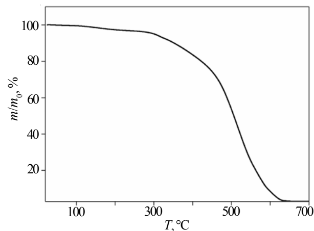
Рис. 4. Данные термогравиметрического анализа ААП
